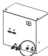
Puesta a tierra consola de dosificación
