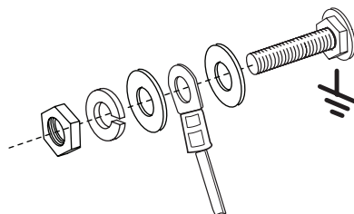
Puesta a tierra consola de ignición
