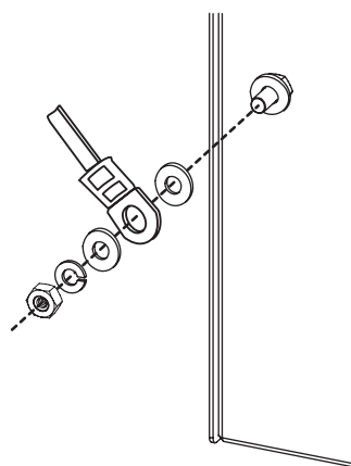
Puesta a tierra consola de selección
