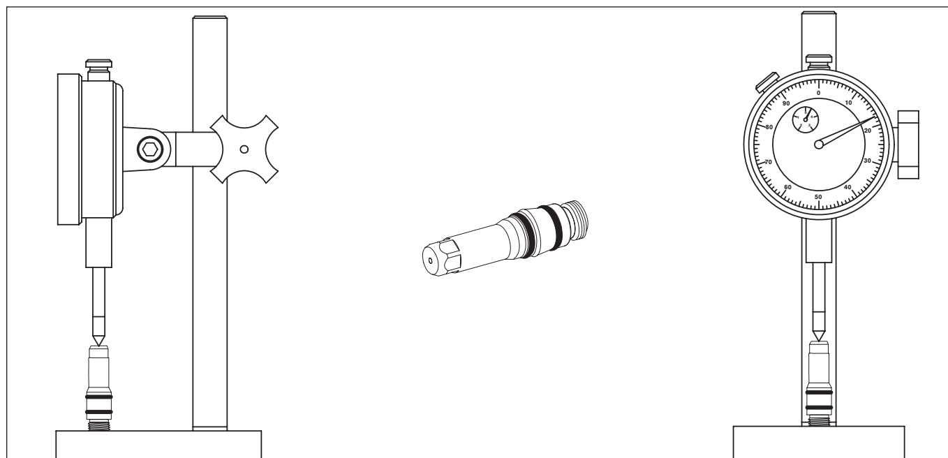
Calibre de profundidad picadura del electrodo (004147)
