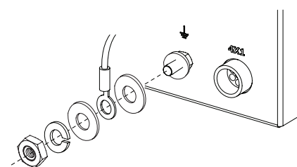
Puesta a tierra consola de dosificación
