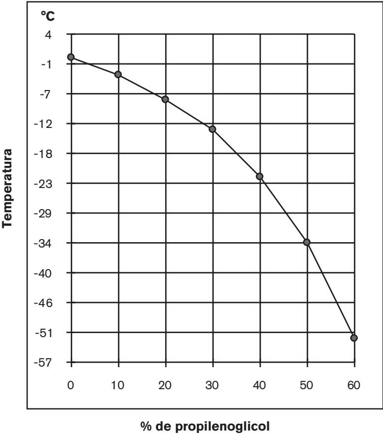
Punto de congelación solución de propilenoglicol
